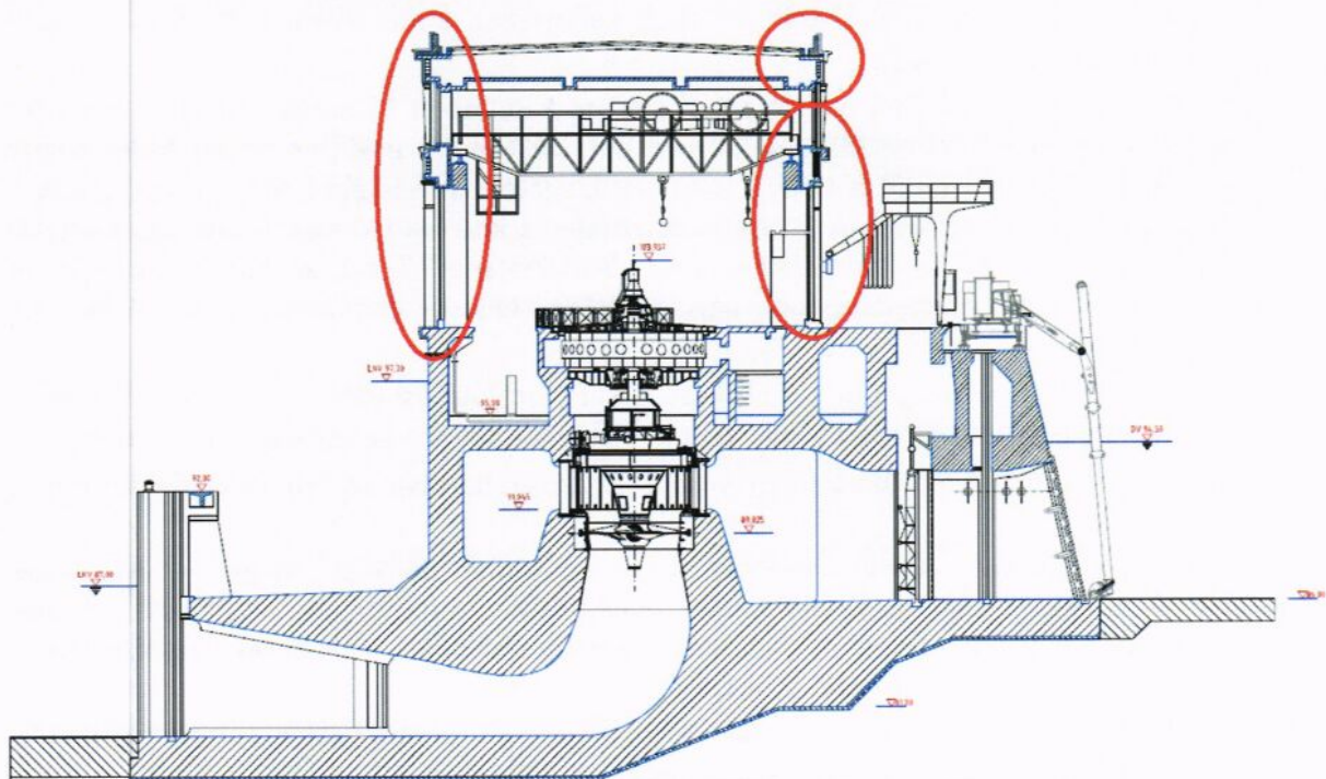
A Tiszalöki Vízerőmű turbina gépház metszete, bejelölve rajta a kivitelezés során fokozott figyelmet és gondosságot igénylő munkaterület részeket.
